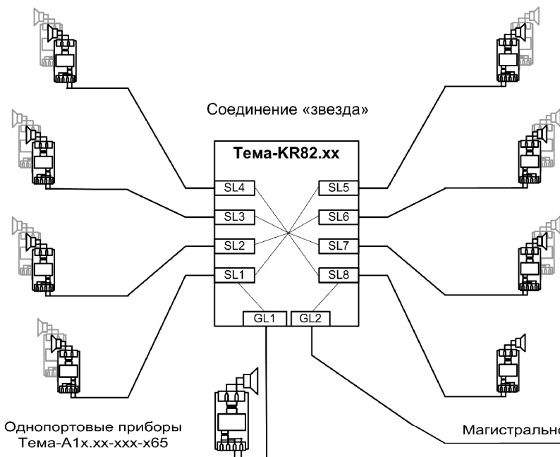
Рис.1. Соединение линий приборов громкоговорящей связи с использованием кросс-коммутатора.
