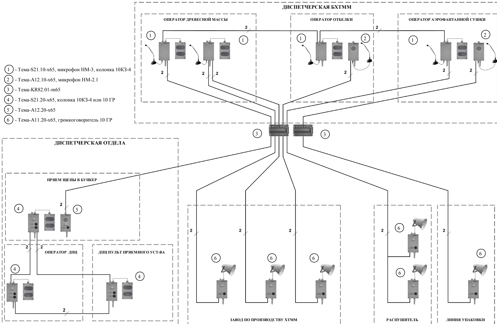
Рис.1. Организация громкоговорящей связи целлюлозно-бумажного комбината.
