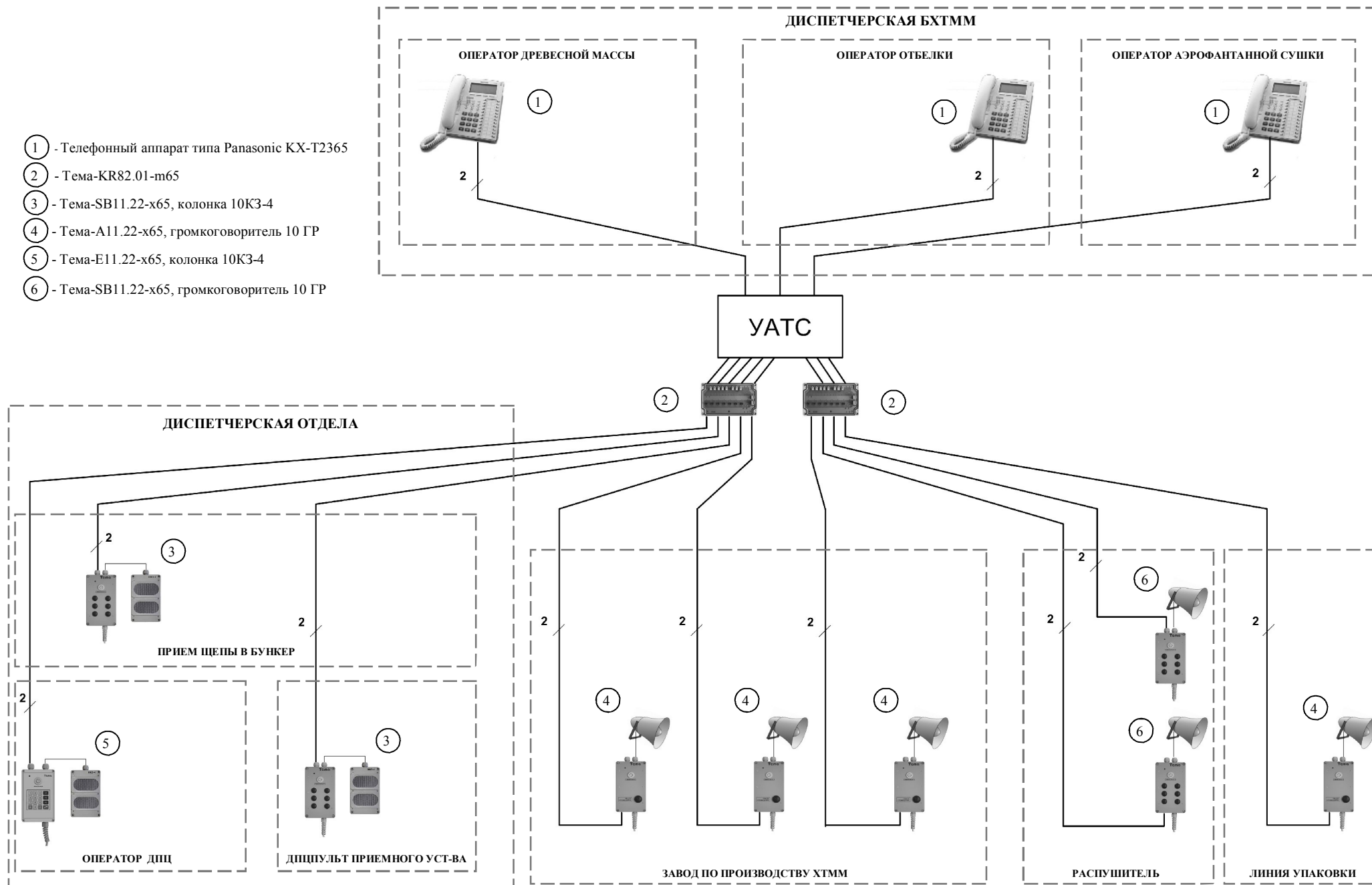
Рис.2. Организация громкоговорящей связи целлюлозно-бумажного комбината на базе УАТС.
