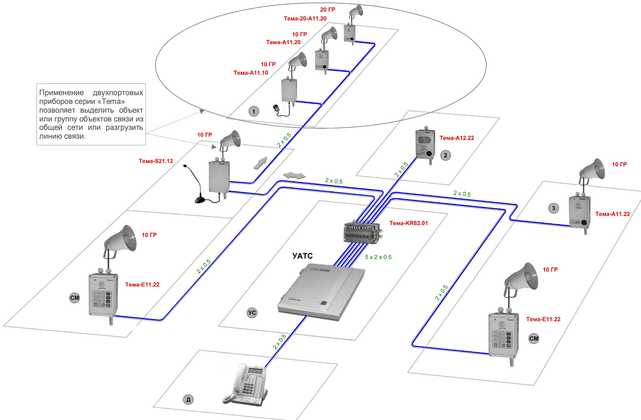
Рис.1. Подключение прибора на два направления к линии громкоговорящей связи и УАТС.
